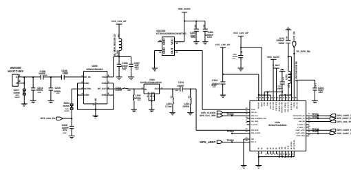
GPS(BCM47511)
